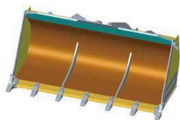
4,5 m³ (Balde con dientes atornillados)
